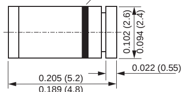
Glass MELF
