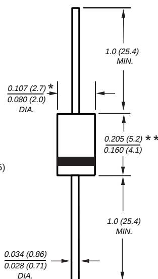
DO-204AL (DO-41)
