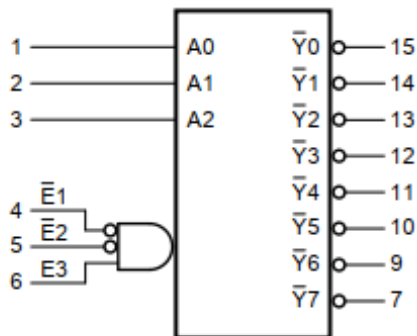
图 1 逻辑符号
