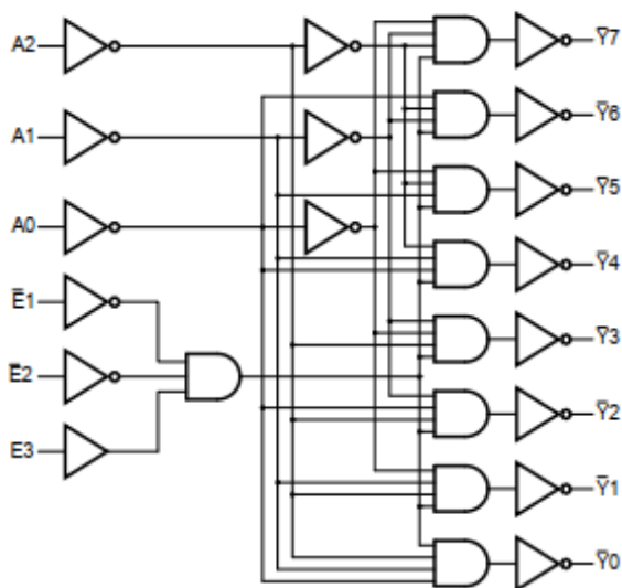
图 3 逻辑框图
